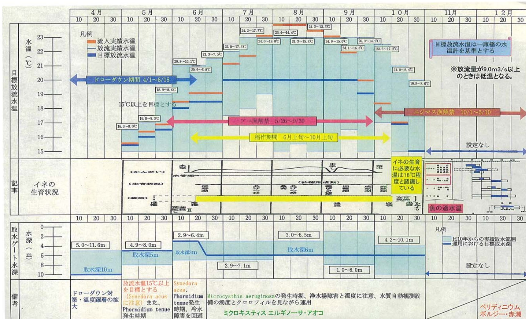
図 8 Fダム選択取水運用ルール
