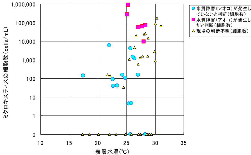
図 4. 12. 14(1) Microcystis 細胞数が年最大時の表層水温と Microcystis 細胞数の関係
